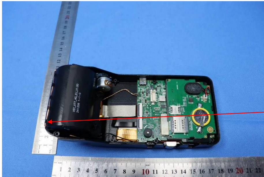
NFC antenna
