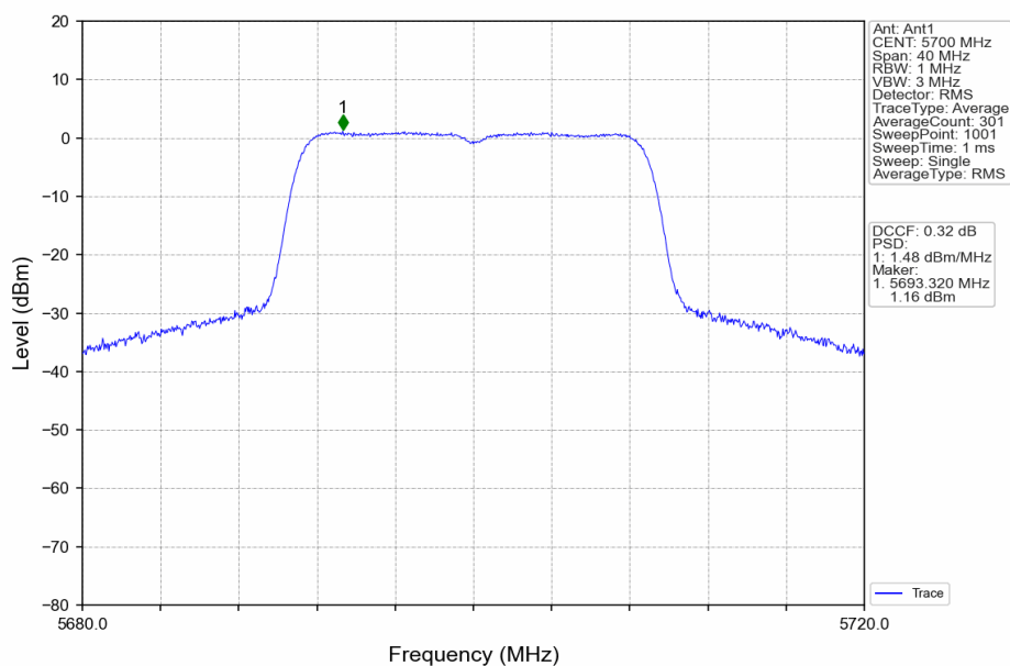
802.11n(HT20)_HCH_5700MHz_Ant1_NTNV
