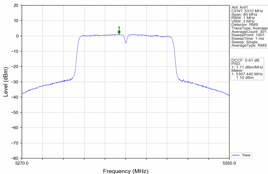
802.11n(HT40)_HCH_5310MHz_Ant1_NTNV
