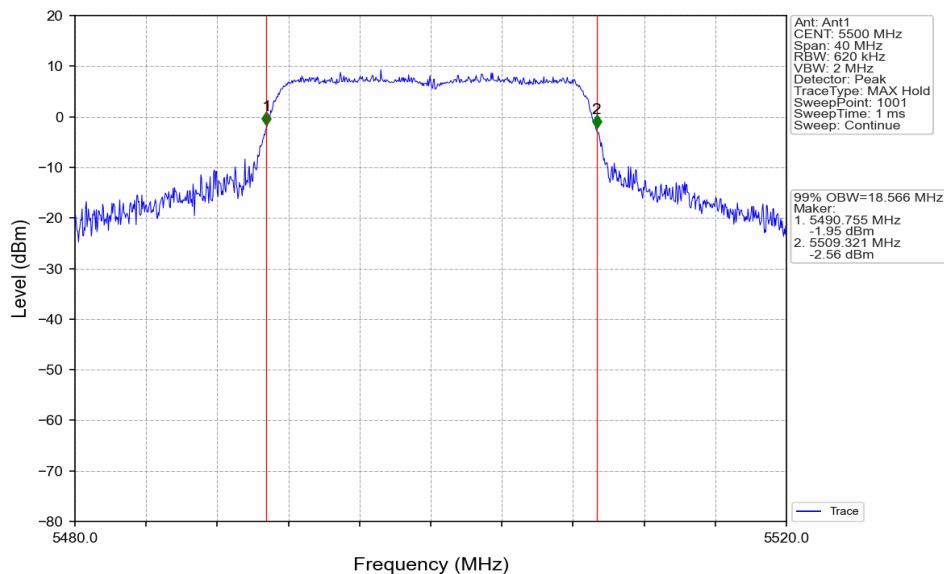
802.11ac(VHT20)_LCH_5500MHz_Ant1_NTNV
