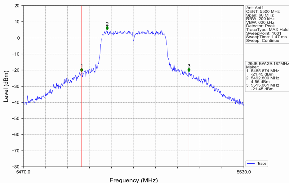
802.11n(HT20)_LCH_5500MHz_Ant1_NTNV
