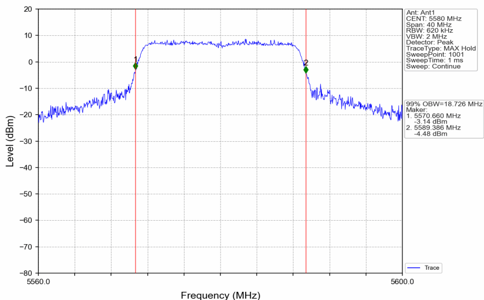
802.11n(HT20)_MCH_5580MHz_Ant1_NTNV
