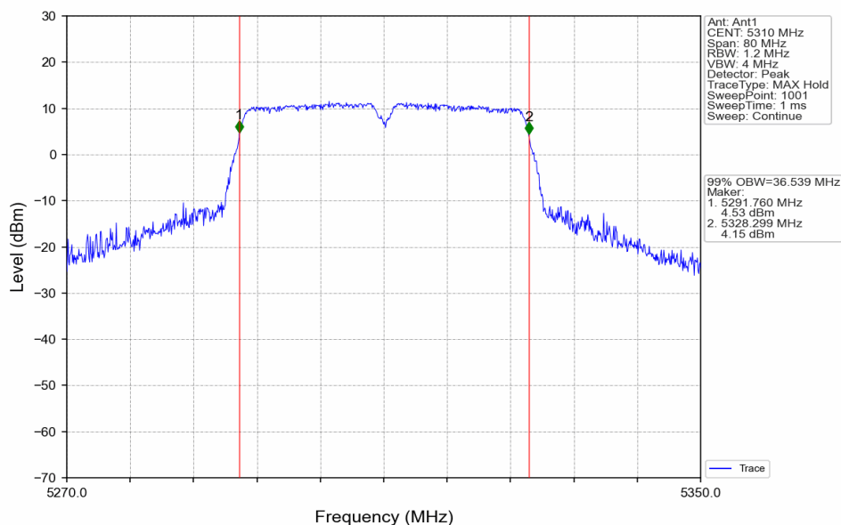
802.11n(HT40)_HCH_5310MHz_Ant1_NTNV
