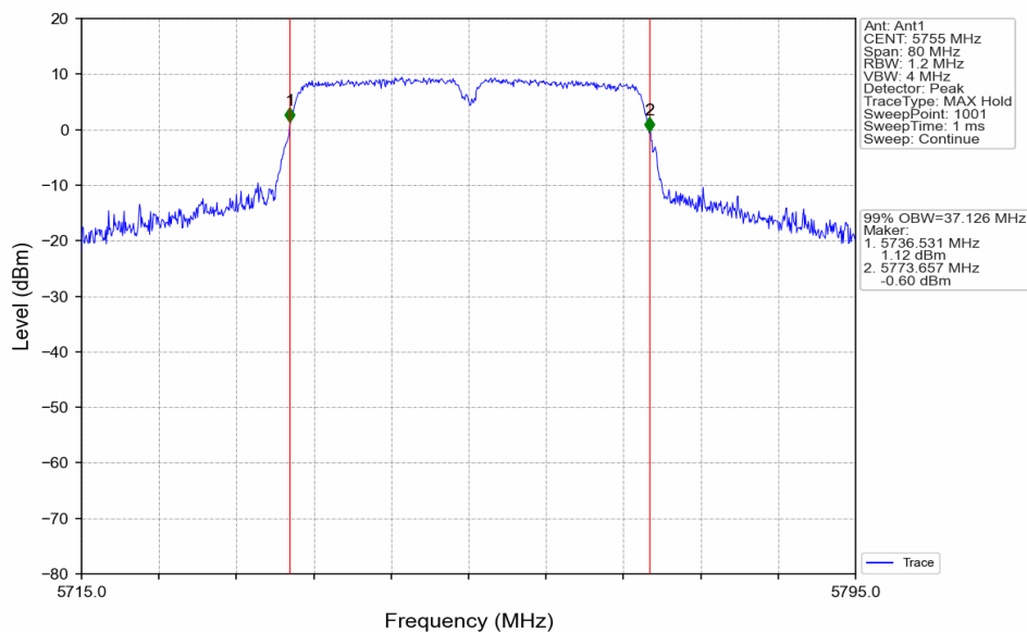
802.11n(HT40)_LCH_5755MHz_Ant1_NTNV
