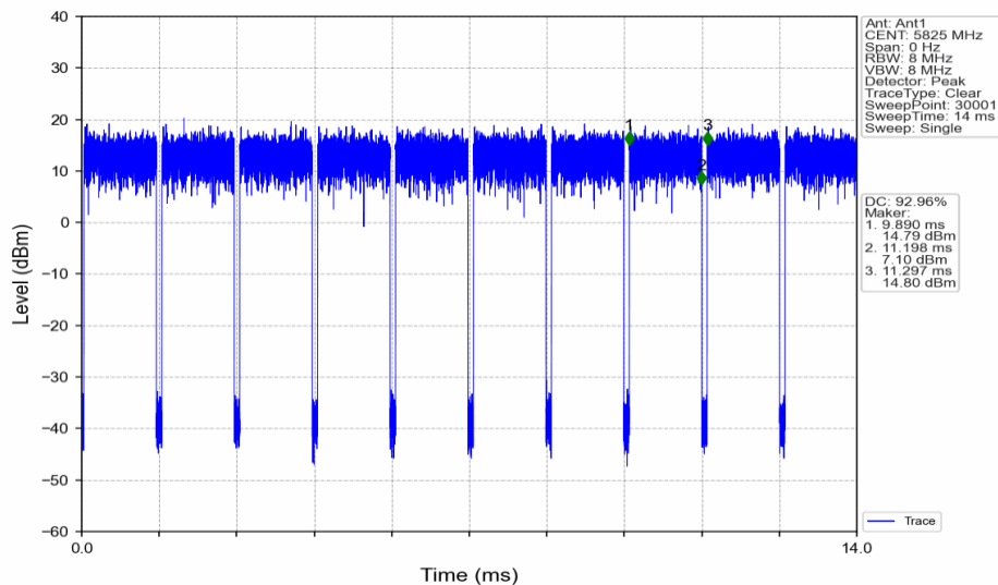
802.11n(HT20)_HCH_5825MHz_Ant1_NTNV
