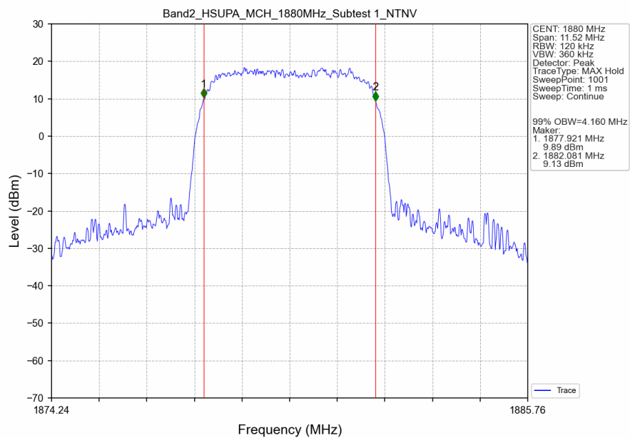
Band2_HSUPA_MCH_1880MHz_Subtest 1_NTNV
