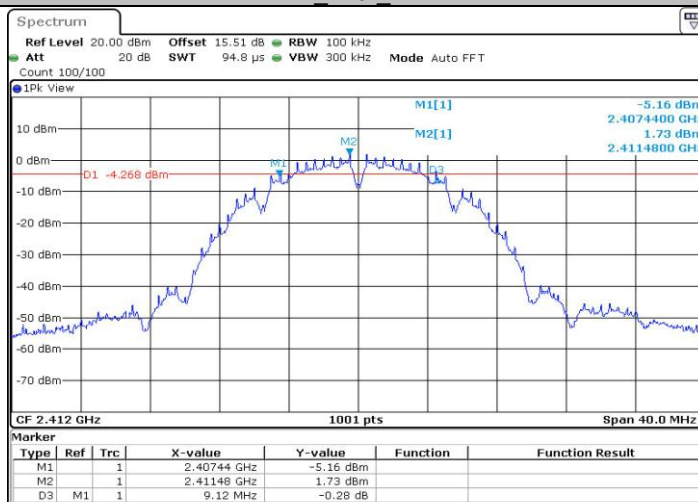
11B_Ant1_2412
