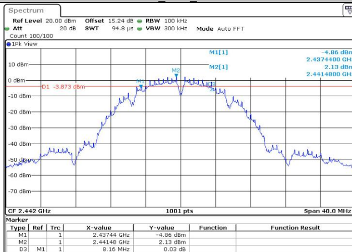
11B_Ant1_2442
