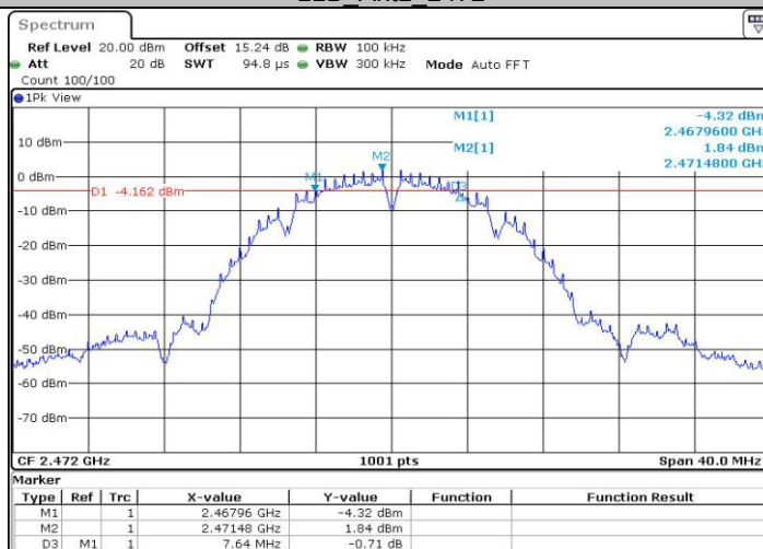
11B_Ant1_2472
