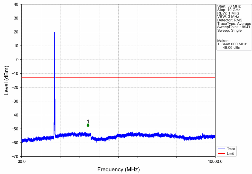
Band4_20MHz_QPSK_MCH_1732.5MHz_RB_1_0_NTNV
