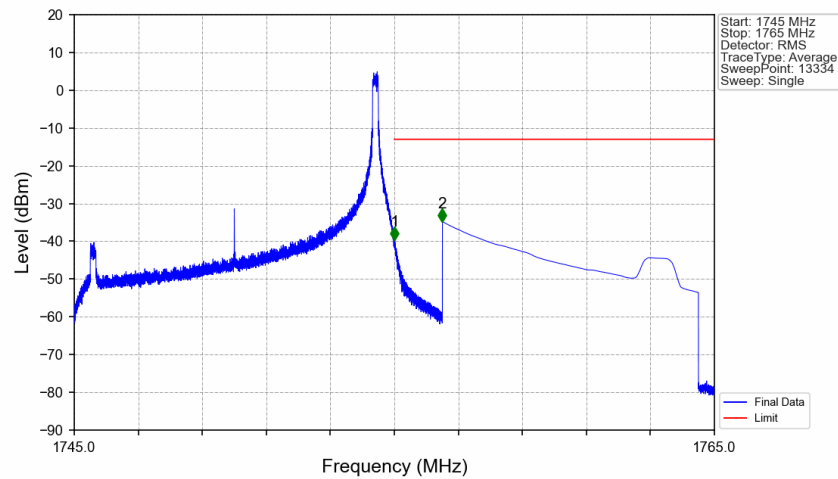
Band4_10MHz_QPSK_HCH_1750MHz_RB_1_49_NTNV
