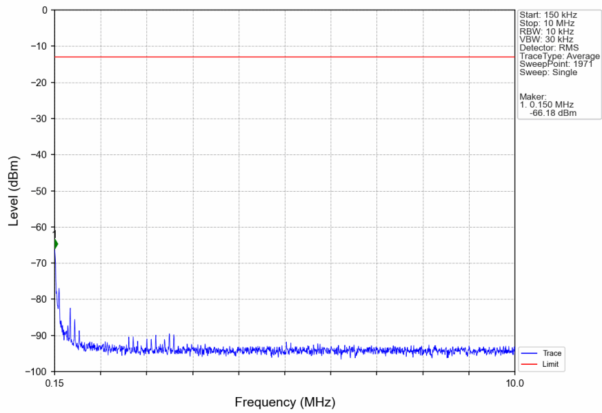
Band4_20MHz_QPSK_MCH_1732.5MHz_RB_1_0_NTNV
