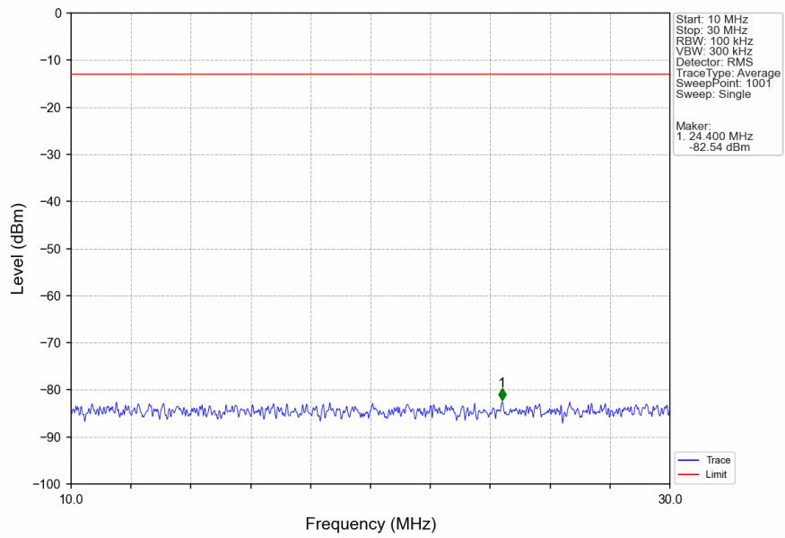
Band4_20MHz_QPSK_HCH_1745MHz_RB_1_0_NTNV
