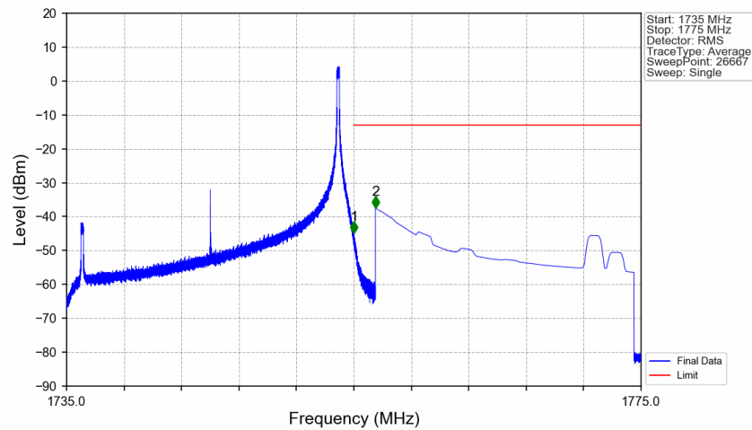
Band4_20MHz_QPSK_HCH_1745MHz_RB_1_99_NTNV
