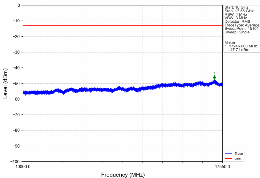
Band4_15MHz_QPSK_HCH_1747.5MHz_RB_1_74_NTNV
