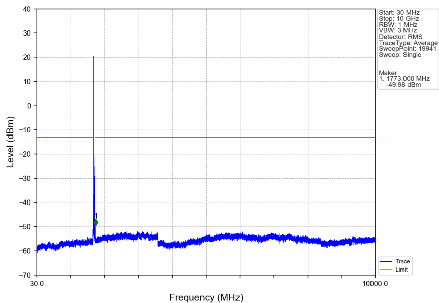
Band4_15MHz_QPSK_LCH_1717.5MHz_RB_1_0_NTNV
