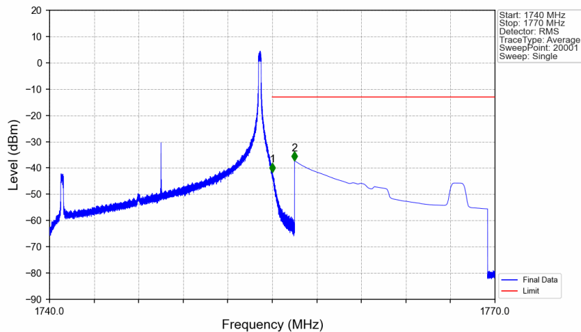
Band4_15MHz_QPSK_HCH_1747.5MHz_RB_1_74_NTNV
