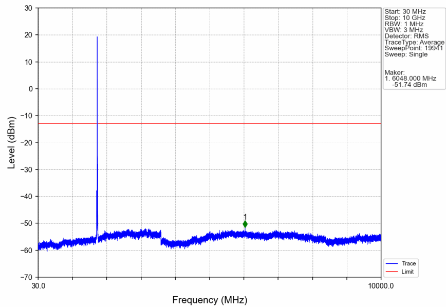
Band4_10MHz_QPSK_HCH_1750MHz_RB_1_0_NTNV
