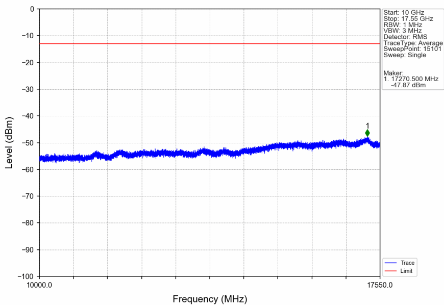
Band4_15MHz_QPSK_LCH_1717.5MHz_RB_1_0_NTNV
