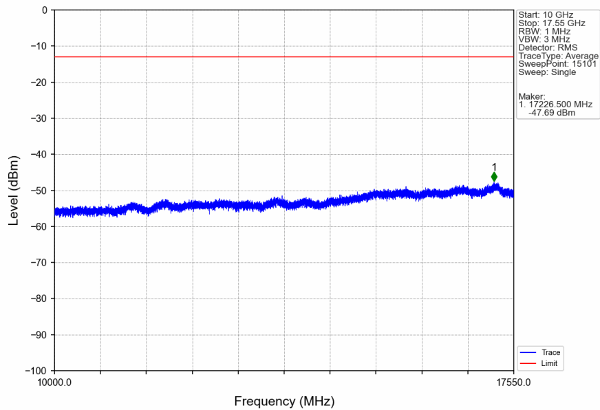
Band4_20MHz_QPSK_HCH_1745MHz_RB_1_99_NTNV
