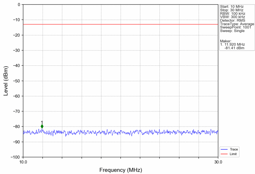
Band4_20MHz_QPSK_LCH_1720MHz_RB_1_0_NTNV
