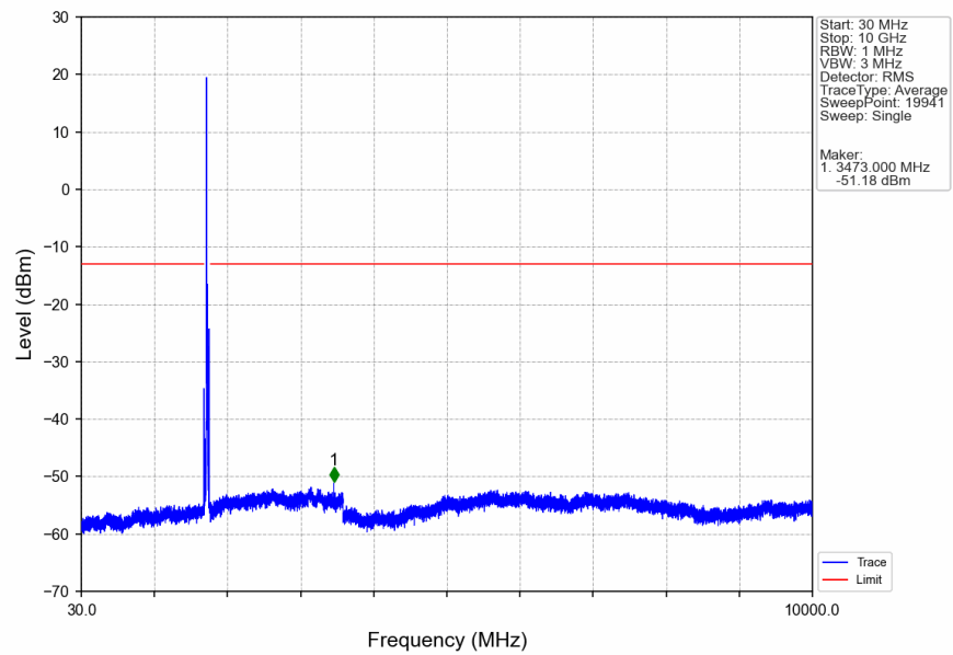
Band4_20MHz_QPSK_HCH_1745MHz_RB_1_0_NTNV
