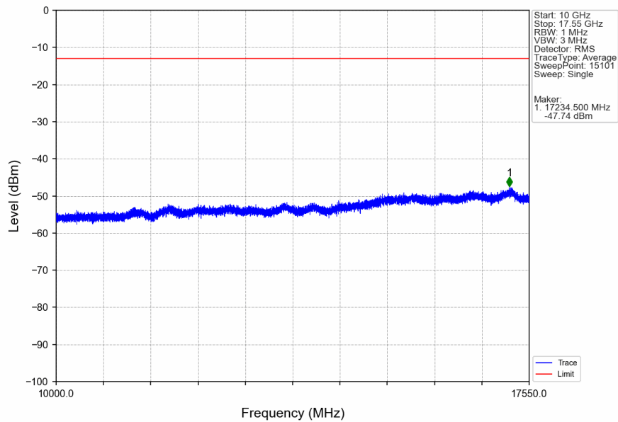
Band4_10MHz_QPSK_HCH_1750MHz_RB_1_49_NTNV
