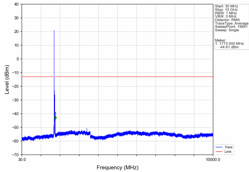
Band4_20MHz_QPSK_LCH_1720MHz_RB_1_0_NTNV
