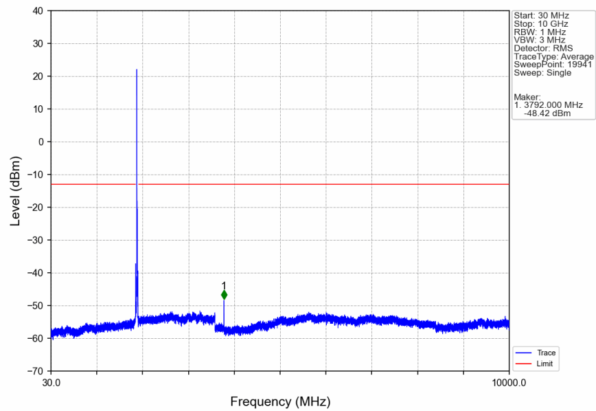
Band2_15MHz_QPSK_HCH_1902.5MHz_RB_1_0_NTNV
