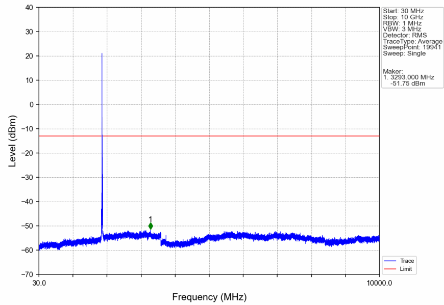
Band2_10MHz_QPSK_MCH_1880MHz_RB_1_0_NTNV
