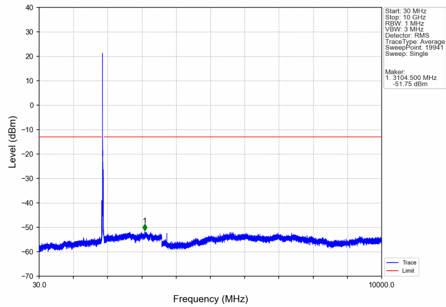
Band2_15MHz_QPSK_MCH_1880MHz_RB_1_0_NTNV
