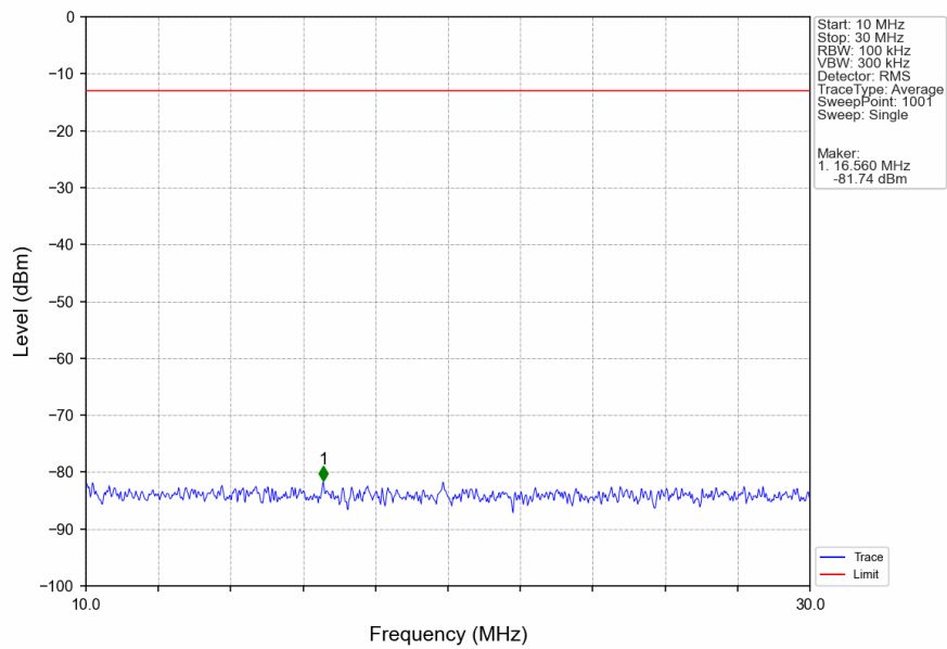
Band2_20MHz_QPSK_LCH_1860MHz_RB_1_0_NTNV
