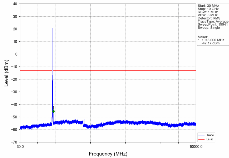
Band2_15MHz_QPSK_LCH_1857.5MHz_RB_1_0_NTNV
