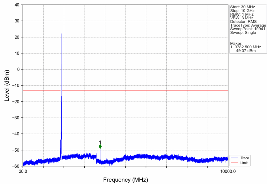
Band2_20MHz_QPSK_HCH_1900MHz_RB_1_0_NTNV
