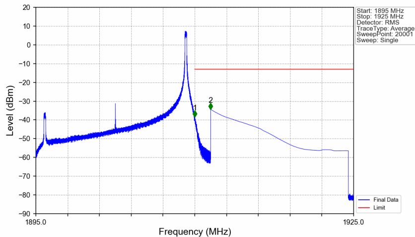
Band2_15MHz_QPSK_HCH_1902.5MHz_RB_1_74_NTNV
