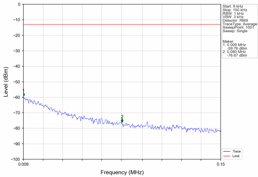
Band2_20MHz_QPSK_HCH_1900MHz_RB_1_0_NTNV
