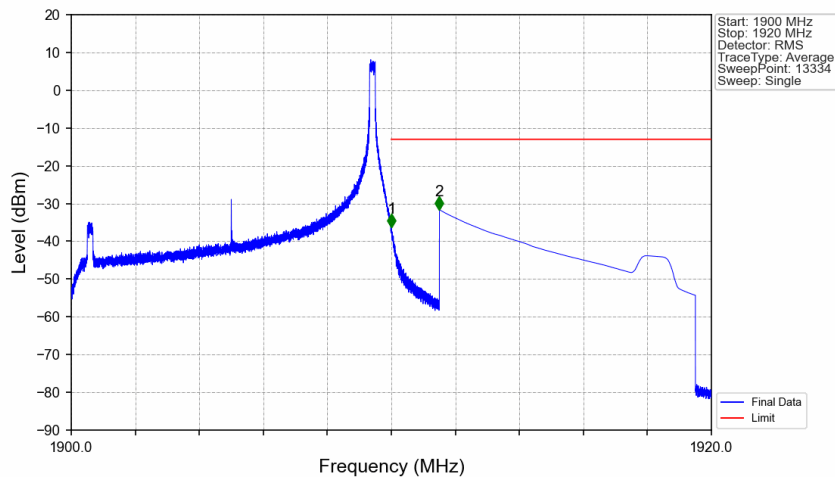
Band2_10MHz_QPSK_HCH_1905MHz_RB_1_49_NTNV
