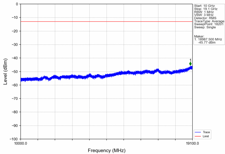
Band2_10MHz_QPSK_MCH_1880MHz_RB_1_0_NTNV
