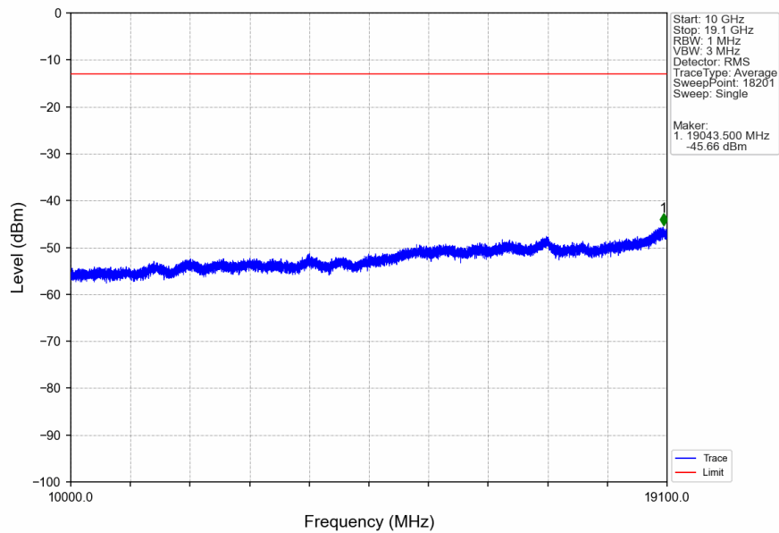
Band2_20MHz_QPSK_HCH_1900MHz_RB_1_99_NTNV
