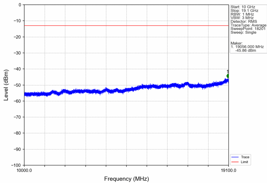
Band2_15MHz_QPSK_LCH_1857.5MHz_RB_1_0_NTNV
