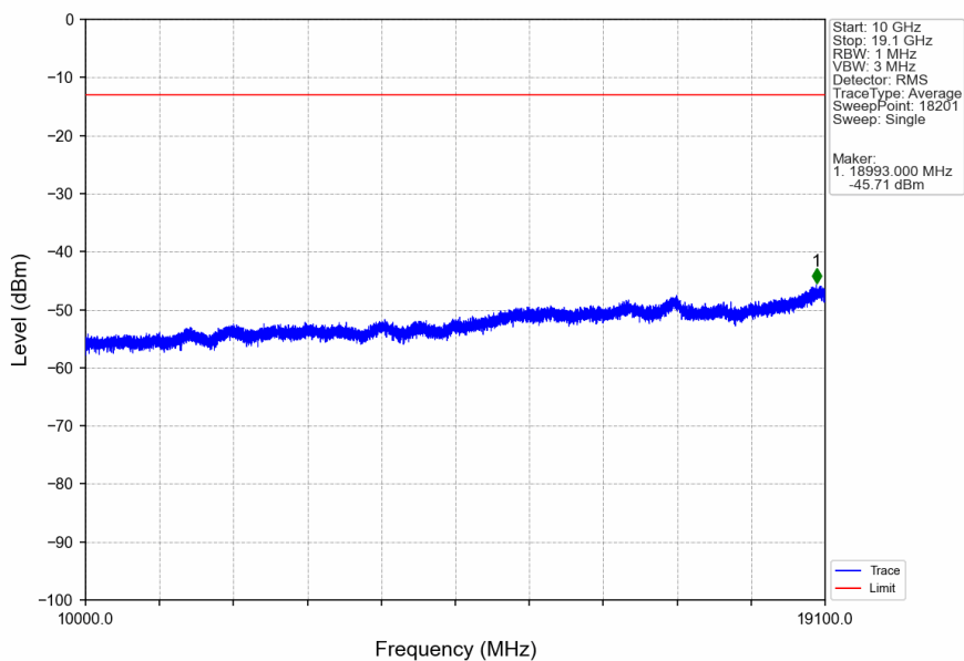
Band2_15MHz_QPSK_HCH_1902.5MHz_RB_1_74_NTNV
