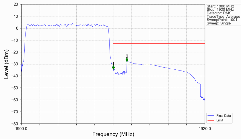
Band2_10MHz_QPSK_HCH_1905MHz_RB_50_0_NTNV
