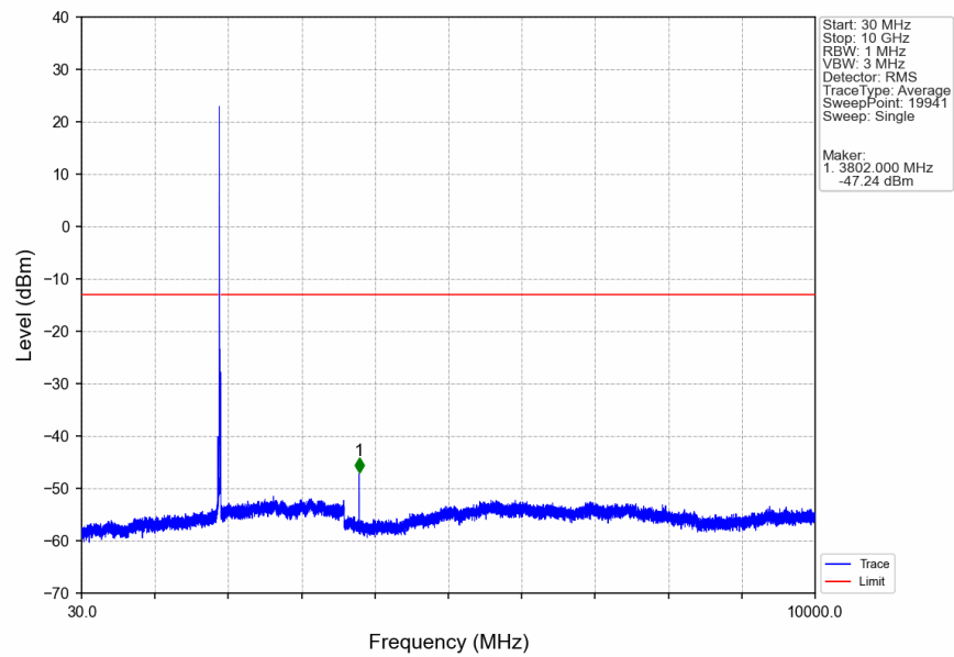
Band2_10MHz_QPSK_HCH_1905MHz_RB_1_0_NTNV
