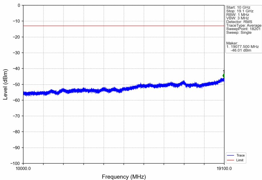
Band2_10MHz_QPSK_HCH_1905MHz_RB_1_49_NTNV
