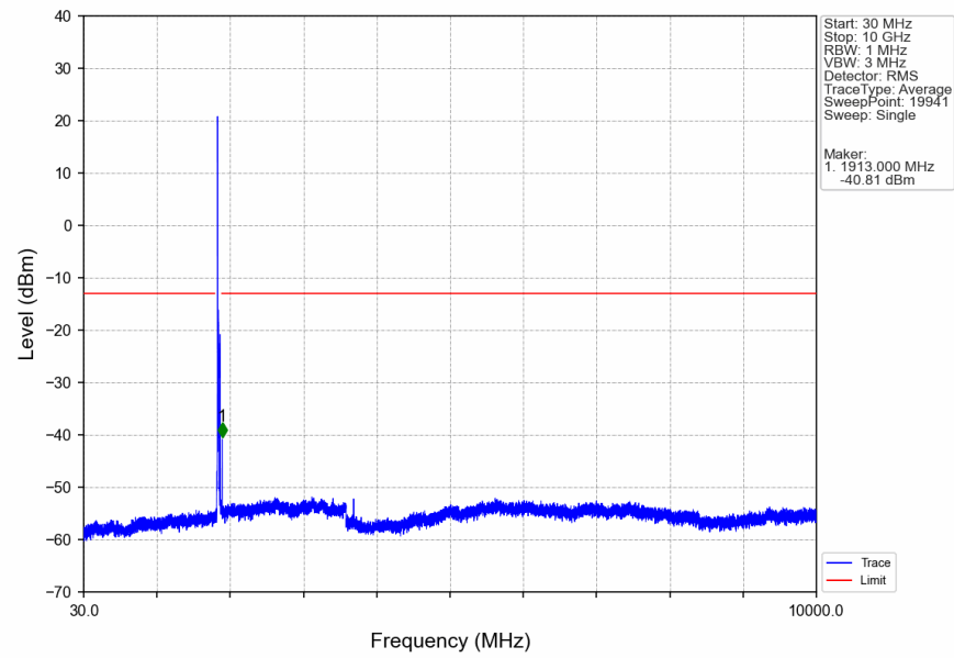
Band2_20MHz_QPSK_LCH_1860MHz_RB_1_0_NTNV
