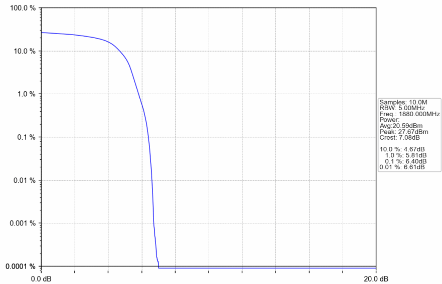
Band2_HSUPA_MCH_1880MHz_Subtest 1_NTNV
