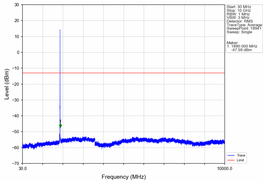
Band2_HSUPA_MCH_1880MHz_Subtest 1_NTNV
