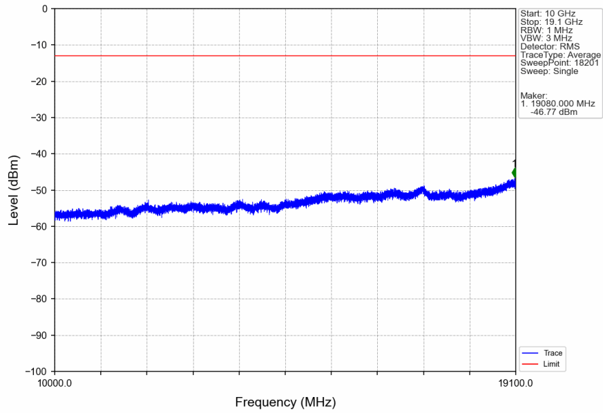
Band2_HSUPA_MCH_1880MHz_Subtest 1_NTNV
