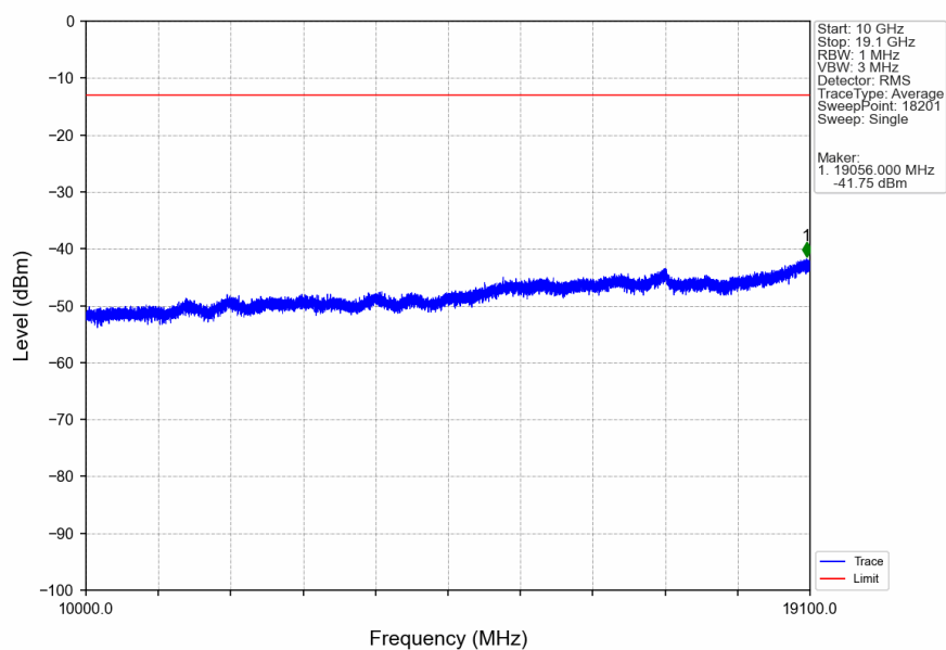
Band2_HSUPA_MCH_1880MHz_Subtest 1_NTNV
