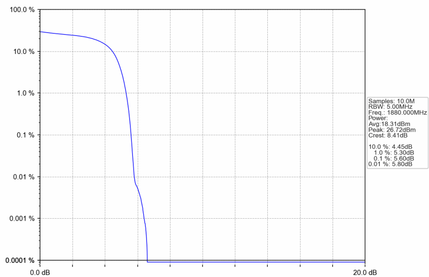
Band2_HSUPA_MCH_1880MHz_Subtest 1_NTNV
