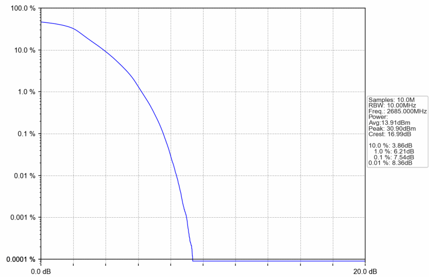
Band41_10MHz_QPSK_HCH_2685MHz_RB_50_0_NTNV
