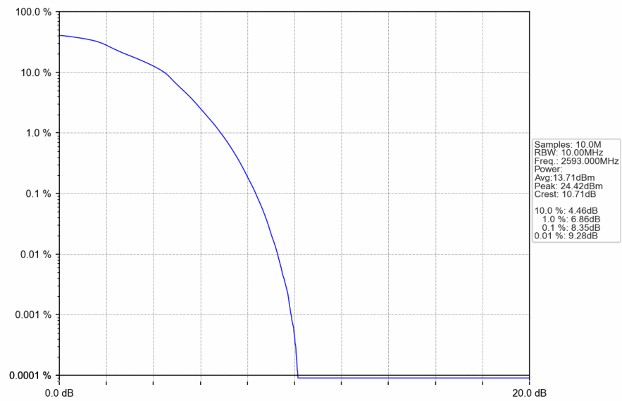
Band41_10MHz_16QAM_MCH_2593MHz_RB_50_0_NTNV
