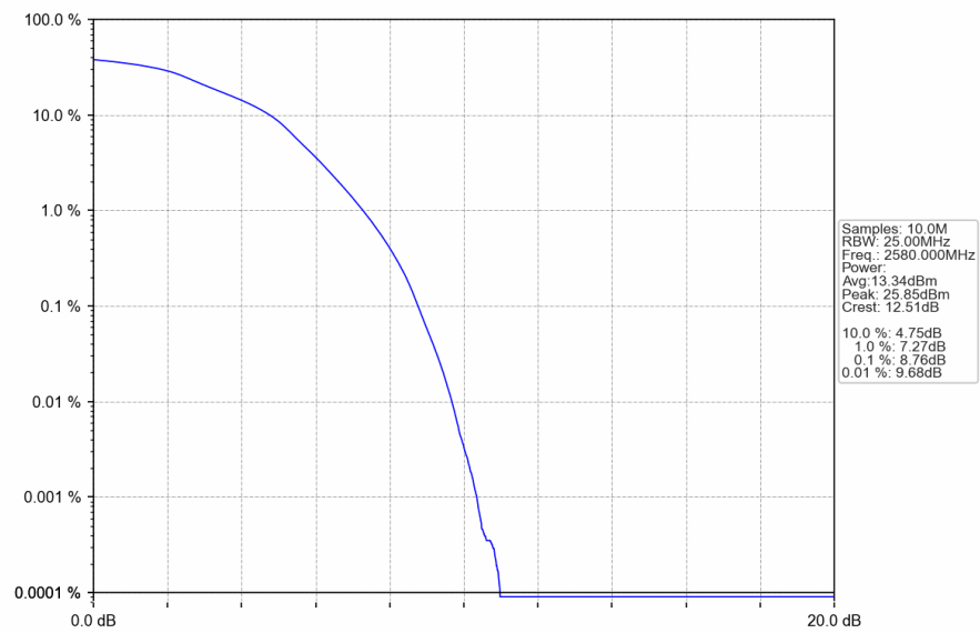
Band38_20MHz_16QAM_LCH_2580MHz_RB_100_0_NTNV
