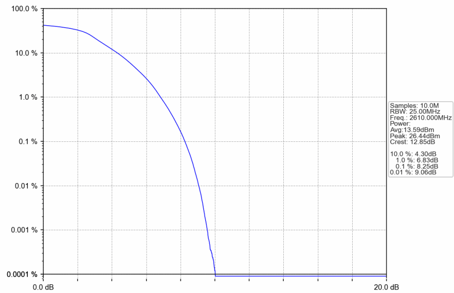
Band38_20MHz_QPSK_HCH_2610MHz_RB_100_0_NTNV
