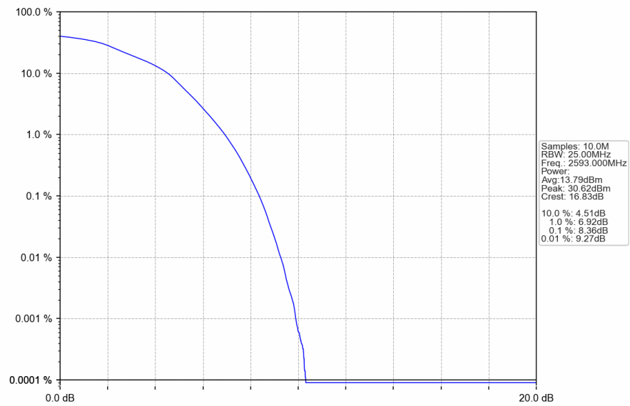
Band41_20MHz_16QAM_MCH_2593MHz_RB_100_0_NTNV
