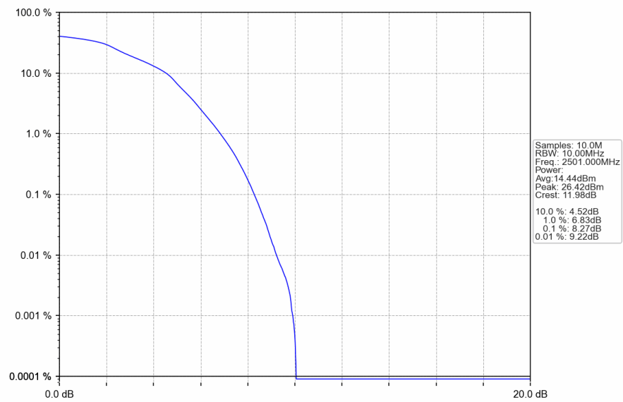
Band41_10MHz_16QAM_LCH_2501MHz_RB_50_0_NTNV
