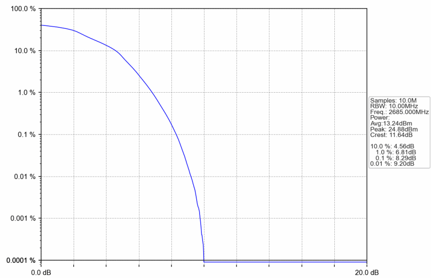
Band41_10MHz_16QAM_HCH_2685MHz_RB_50_0_NTNV
