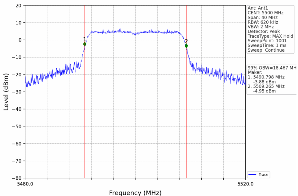
802.11ac(VHT20)_LCH_5500MHz_Ant1_NTNV
