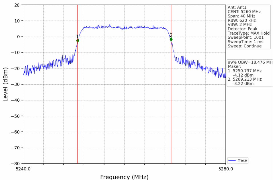
802.11n(HT20)_LCH_5260MHz_Ant1_NTNV
