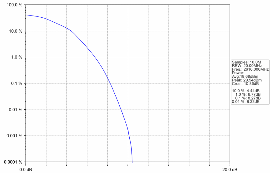
Band38_20MHz_16QAM_HCH_2610MHz_RB_100_0_NTNV
