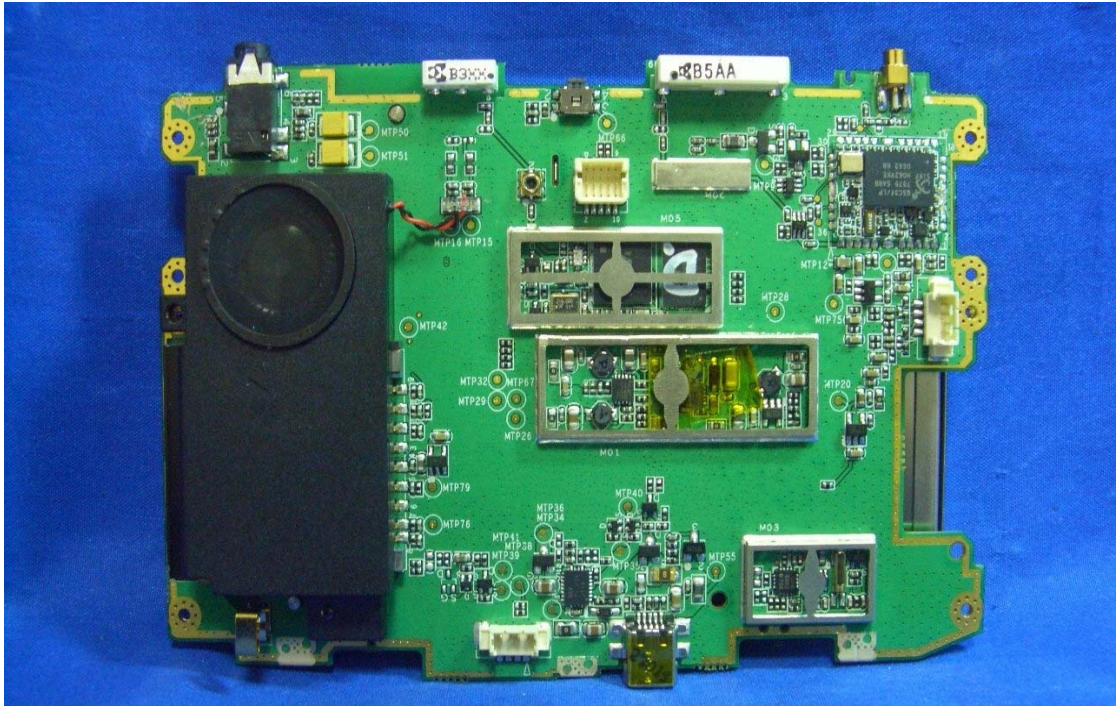
(13) EUT Photo
