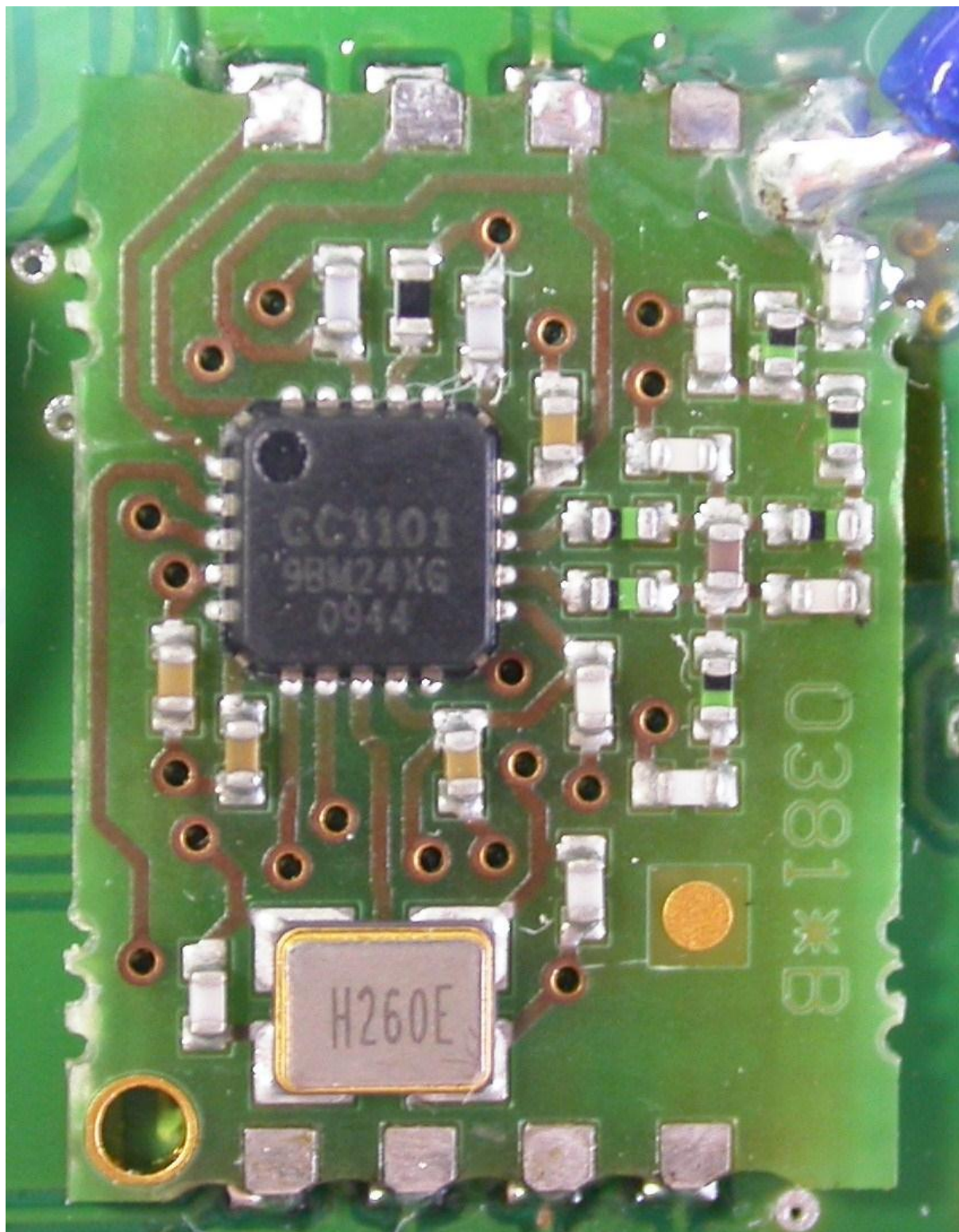
RF module top view (zoom)
