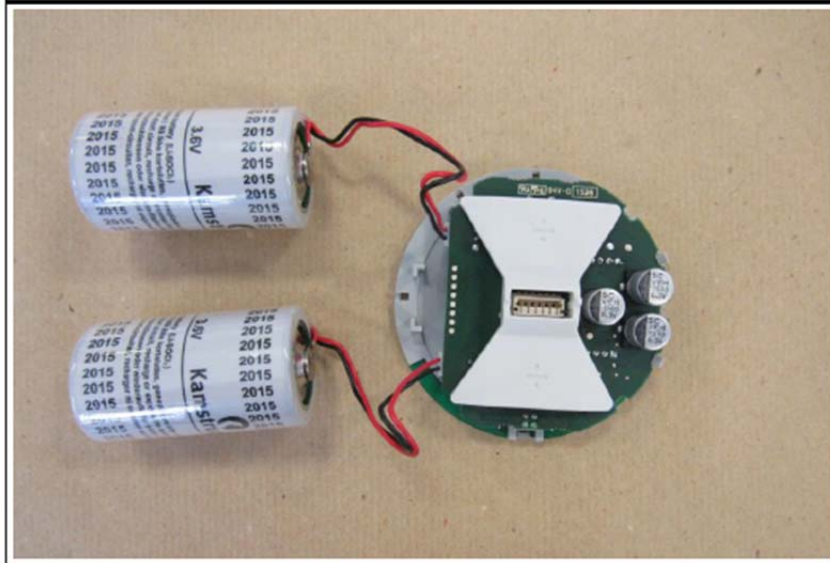
EUT PCB II back I
