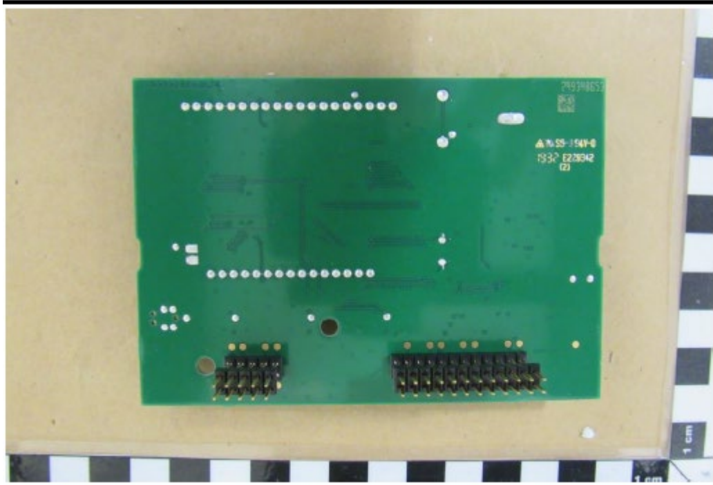
MULTICAL® 603 PCB BOTTOM SIDE
