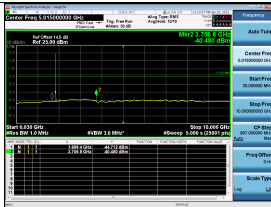
B25-10M-Mid CH-CSE-2-Q16-1 RB 0
