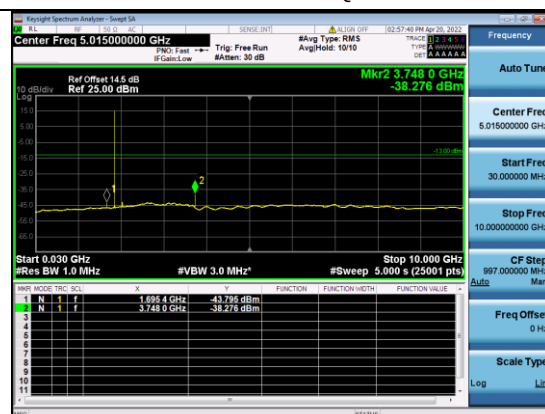
B25-20M-Mid CH-CSE-2-Q16-1 RB 0
