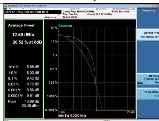
B12-5M-Low CH-PAPR-QPSK
