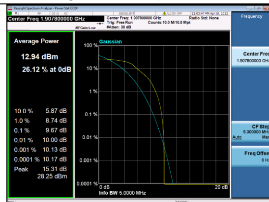
B2-3M-High CH-PAPR-Q16
