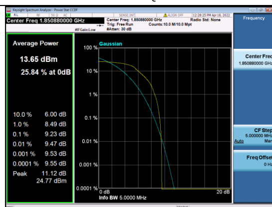
B2-5M-Low CH-PAPR-QPSK
