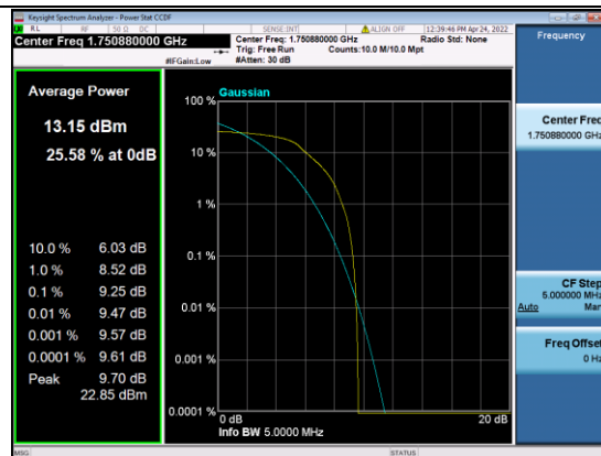
B4-5M-Low CH-PAPR-QPSK
