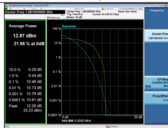
B25-3M-Mid CH-PAPR-Q16
