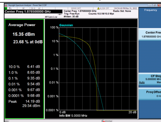
B25-15M-Mid CH-PAPR-Q16
