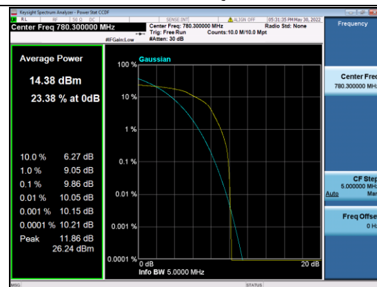
B13-5M-Mid CH-PAPR-Q16
