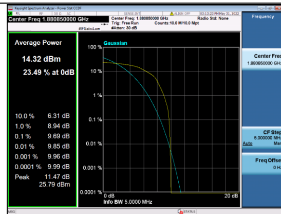
B25-5M-Mid CH-PAPR-Q16
