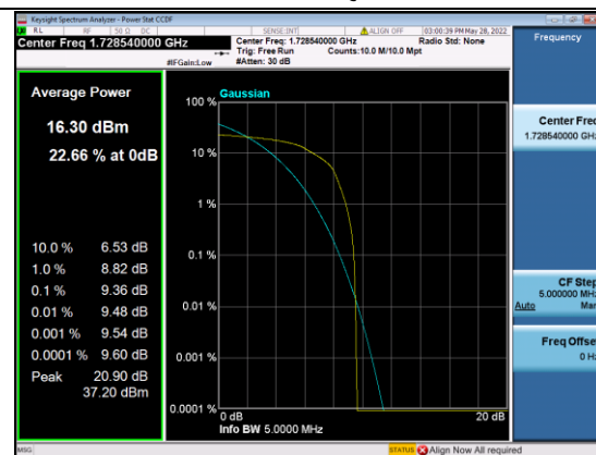
B4-10M-Mid CH-PAPR-Q16
