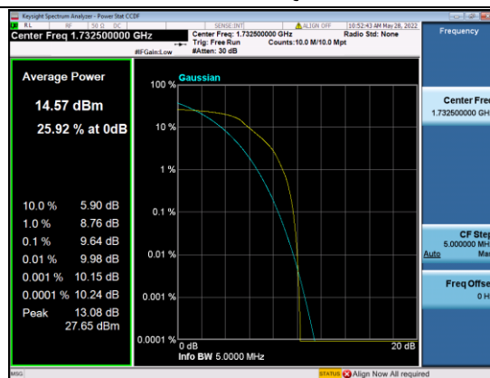
B4-1.4M-Mid CH-PAPR-QPSK
