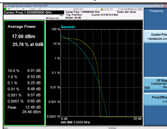
B2-5M-Mid CH-PAPR-QPSK
