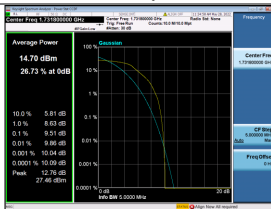
B4-3M-Mid CH-PAPR-QPSK
