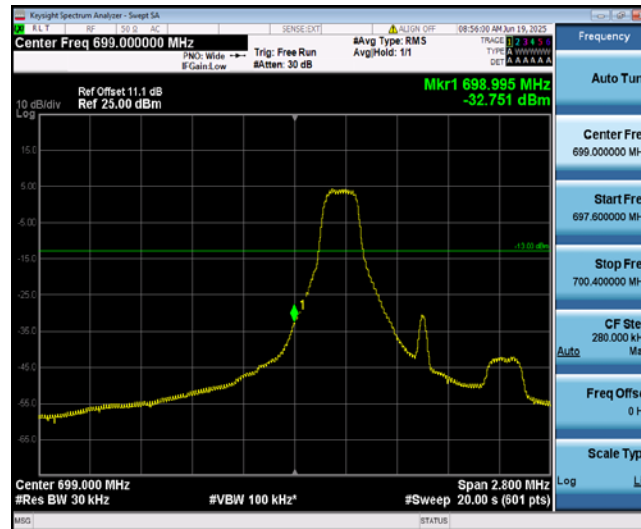
Band12-1.4MHz-QPSK-23017-1-0-Low--32.75-PASS
