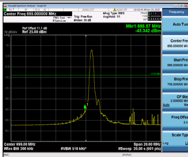
Band12-10MHz-QPSK-23060-1-0-Low--45.34-PASS
