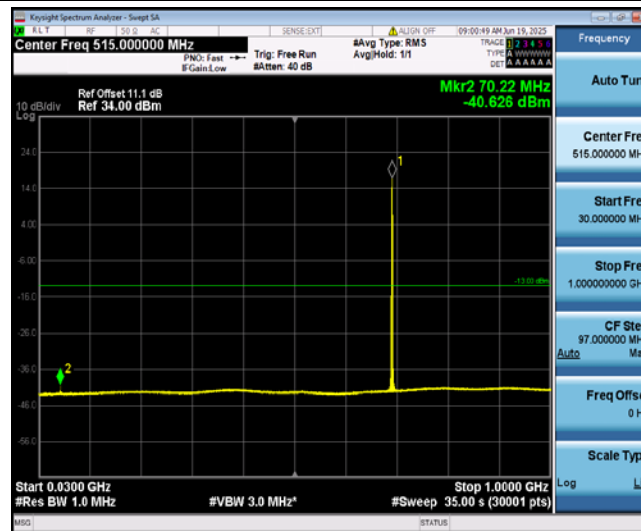
Band12-1.4MHz-QPSK-23017-1-0-Low-30-1000--40.63-PASS
