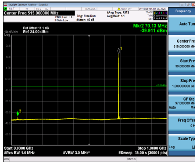
Band12-3MHz-QPSK-23025-1-0-Low-30-1000--39.91-PASS
