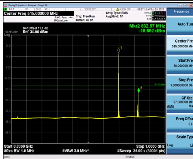
Band12-1.4MHz-QPSK-23095-1-0-Low-30-1000--19.69-PASS
