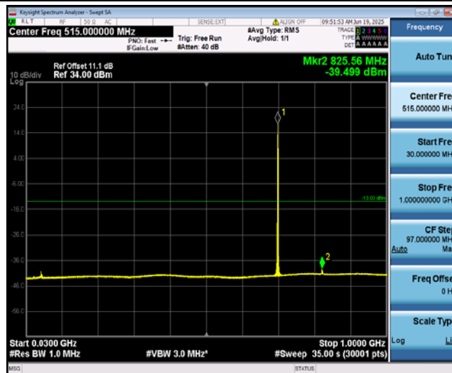
Band12-3MHz-QPSK-23095-1-0-Low-30-1000--39.5-PASS
