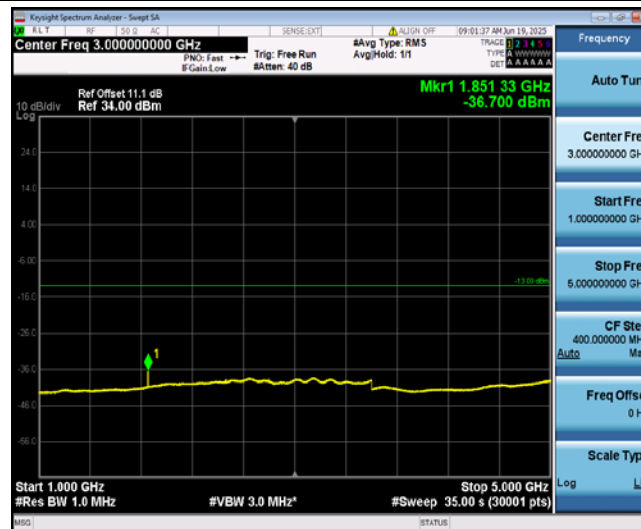
Band12-1.4MHz-QPSK-23017-1-0-Low-1000-5000--36.7-PASS
