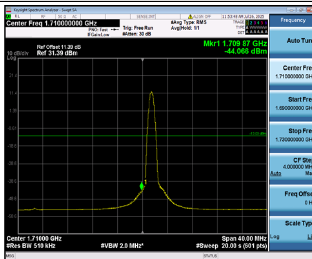
Band4-20MHz-16QAM-20050-1-0-Low--44.07-PASS
