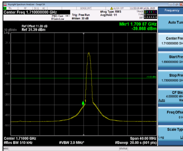
Band4-20MHz-QPSK-20050-1-0-Low--39.87-PASS
