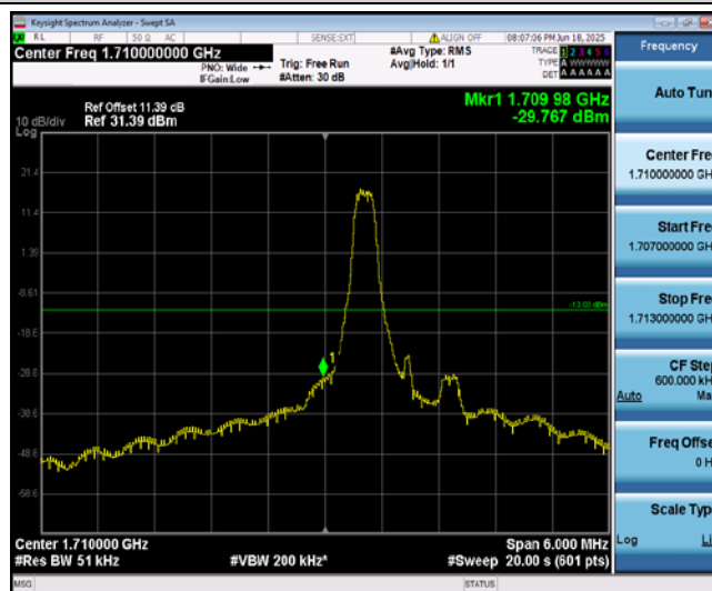
Band4-3MHz-QPSK-19965-1-0-Low--29.77-PASS
