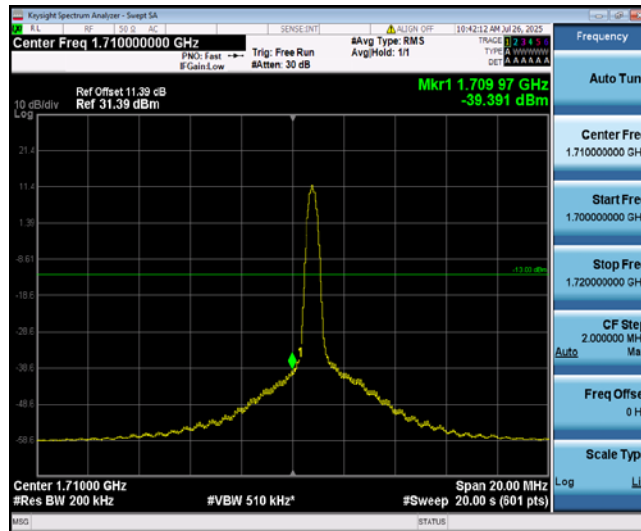
Band4-10MHz-QPSK-20000-1-0-Low--39.39-PASS
