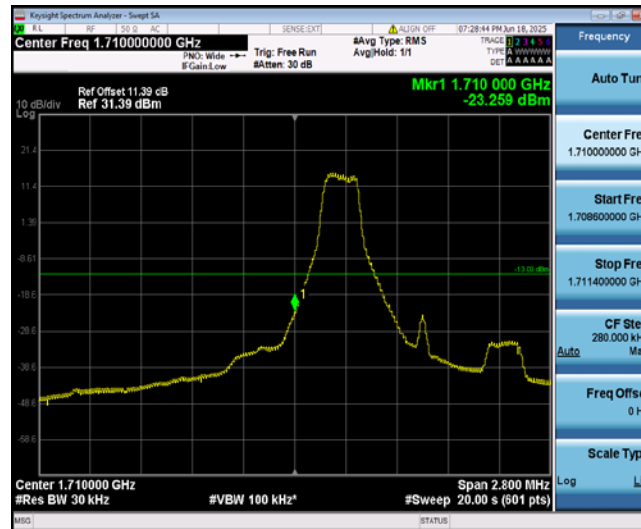
Band4-1.4MHz-QPSK-19957-1-0-Low--23.26-PASS
