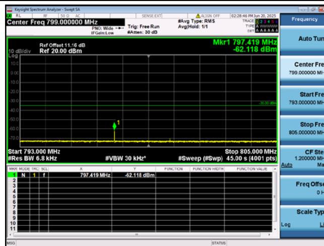
Band13-10MHz-QPSK-23230-1-0-Middle--62.118-PASS
