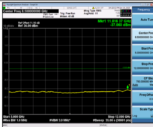
Band13-5MHz-QPSK-23230-1-0-Low-5000-12000--37.06-PASS
