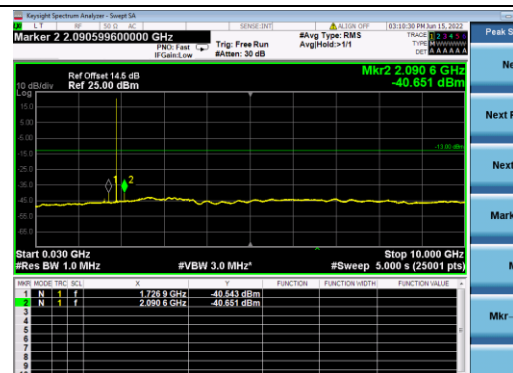
B2-20M-High CH-CSE-2-Q16-1 RB 0
