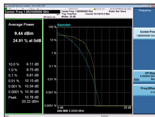
B25-1.4M-Mid CH-PAPR-Q16
