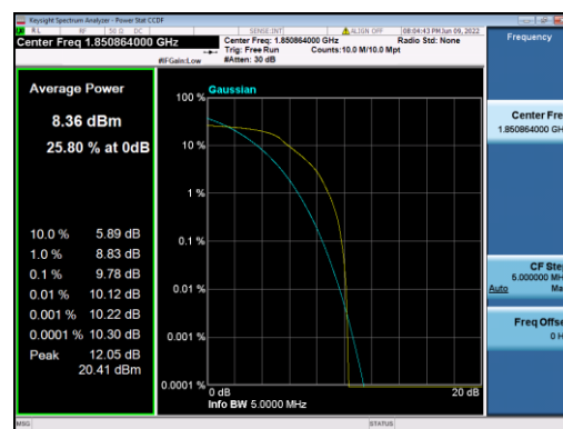
B25-3M-Mid CH-PAPR-QPSK
