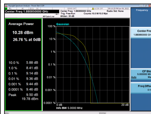
B25-5M-Mid CH-PAPR-QPSK
