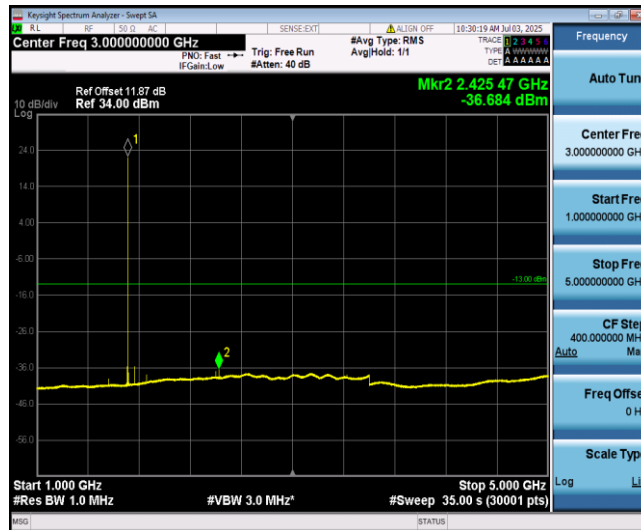
Band66-20MHz-QPSK-132072-1-0-Low-1000-5000--36.68-PASS
