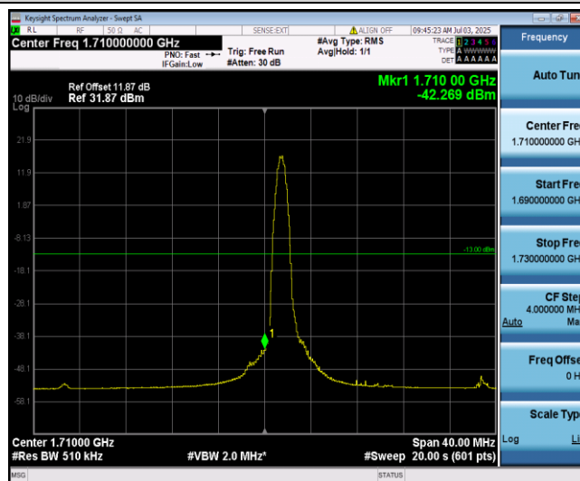
Band66-20MHz-16QAM-132072-1-0-Low--42.27-PASS
