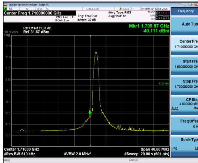
Band66-20MHz-QPSK-132072-1-0-Low--40.11-PASS
