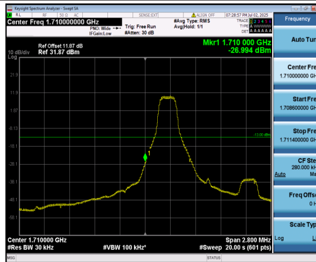
Band66-1.4MHz-QPSK-131979-1-0-Low--26.99-PASS
