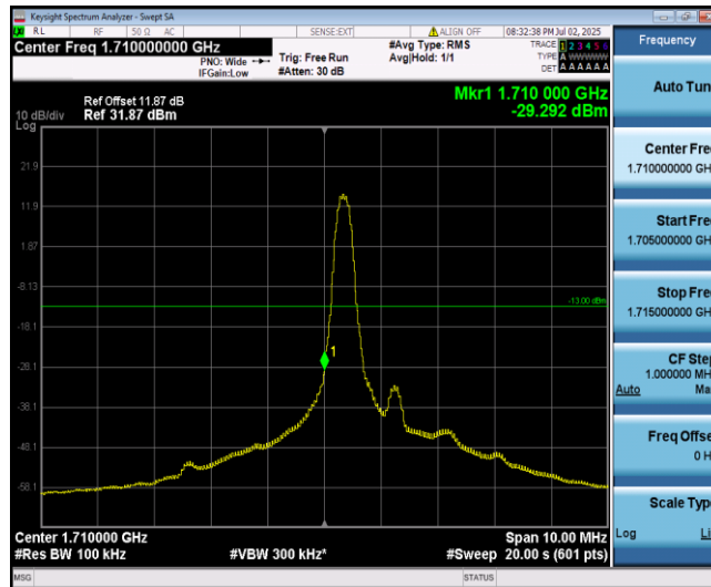
Band66-5MHz-QPSK-131997-1-0-Low--29.29-PASS
