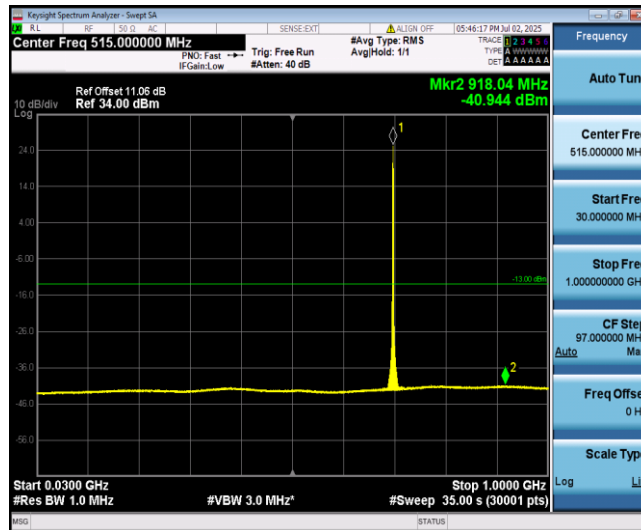
Band12-5MHz-QPSK-23095-1-0-Low-30-1000--40.94-PASS
