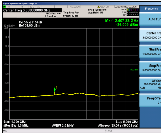
Band12-1.4MHz-16QAM-23017-1-0-Low-1000-5000--36.01-PASS
