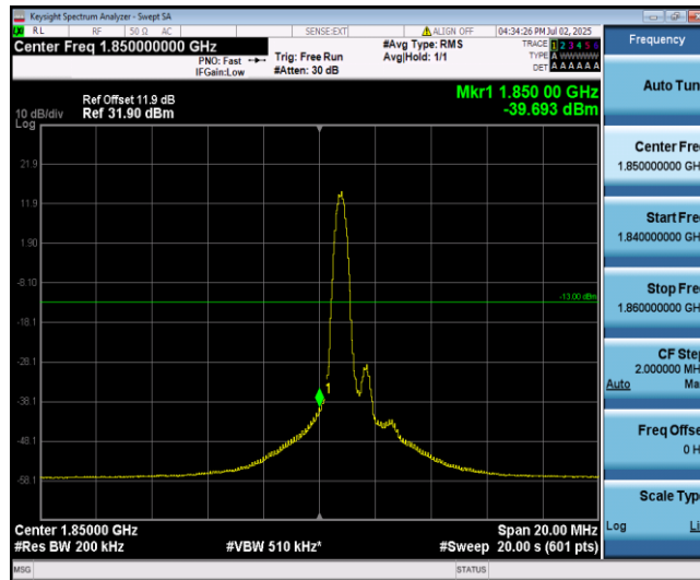
Band2-10MHz-QPSK-18650-1-0-Low--39.69-PASS
