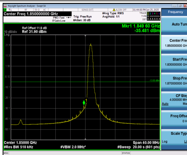
Band2-20MHz-16QAM-18700-1-0-Low--35.48-PASS
