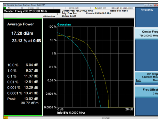
B13-5M-Low CH-PAPR-Q16
