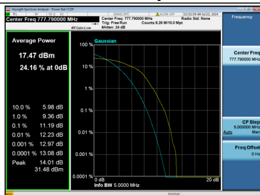
B13-5M-Mid CH-PAPR-Q16
