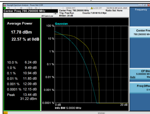
B13-5M-Mid CH-PAPR-QPSK
