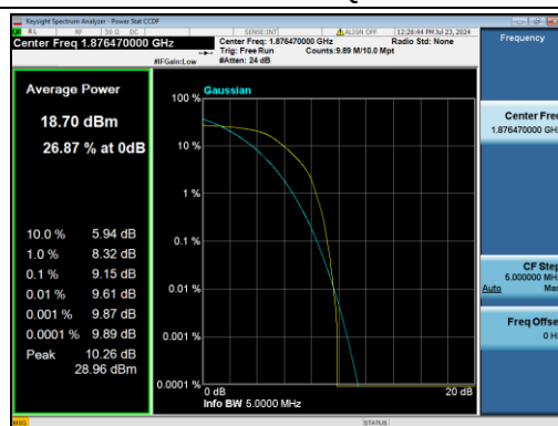
B25-15M-Mid CH-PAPR-QPSK
