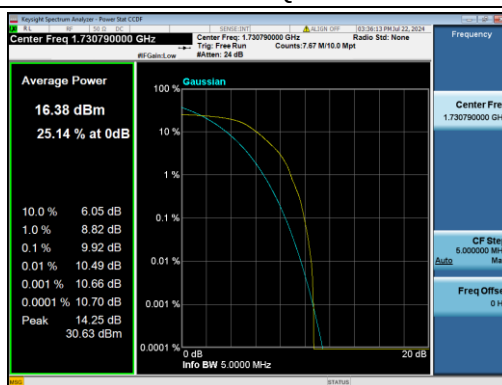
B4-5M-Mid CH-PAPR-QPSK
