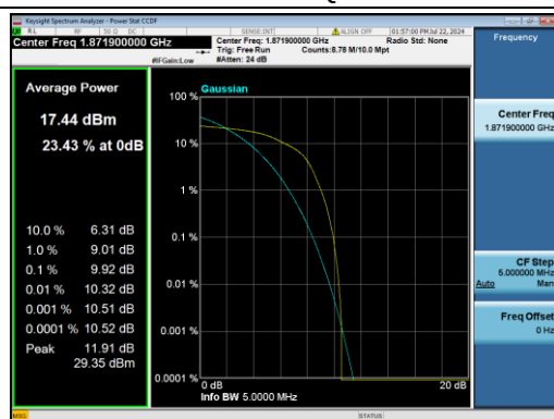
B2-20M-Mid CH-PAPR-Q16
