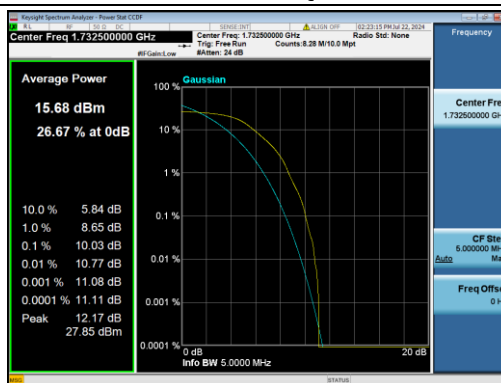
B4-1.4M-Mid CH-PAPR-QPSK
