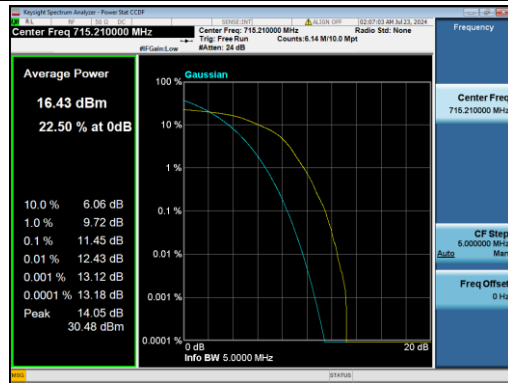
B12-5M-Low CH-PAPR-Q16
