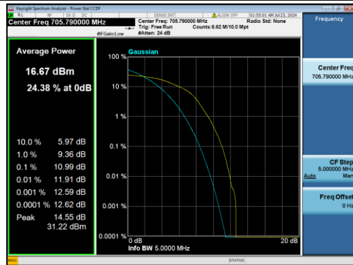
B12-5M-Mid CH-PAPR-Q16
