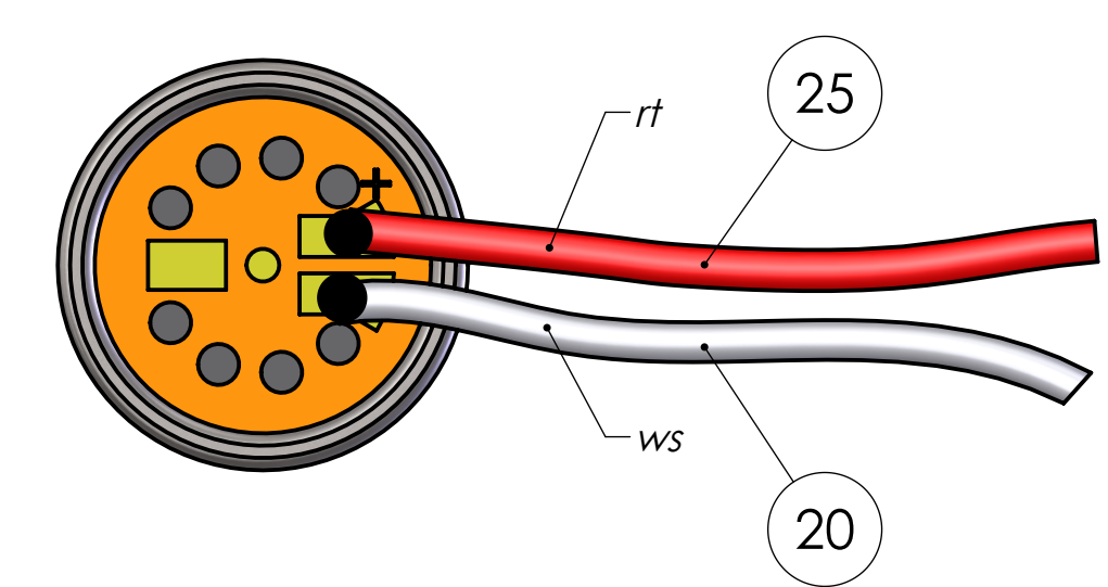
Lötansicht von Pos (75)
