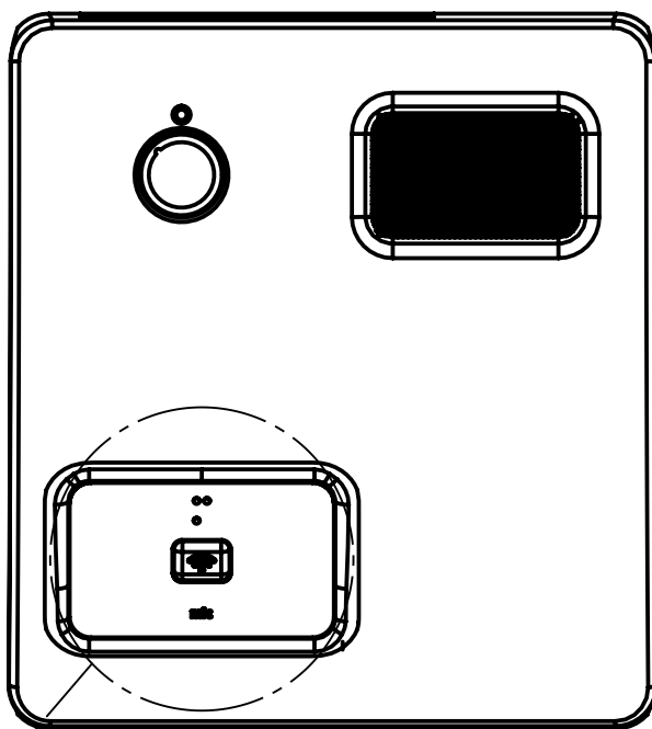
DETAIL Z 1:1
