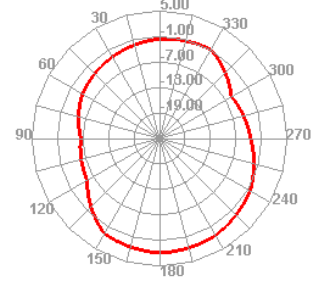
2440.000MHz H
