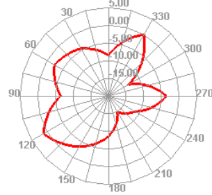
2440.000MHz E2
