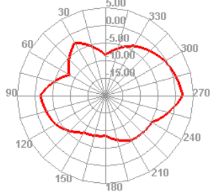
2440.000MHz E1
