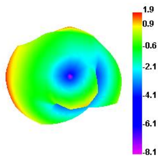
2440.000MHz
