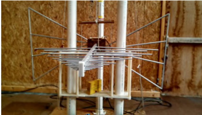
3142 Biconilog Antenna
