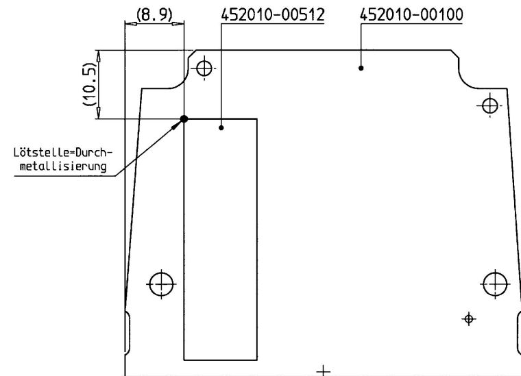
Ansicht Top Layer mit Schirmfolie (vereinfacht)
