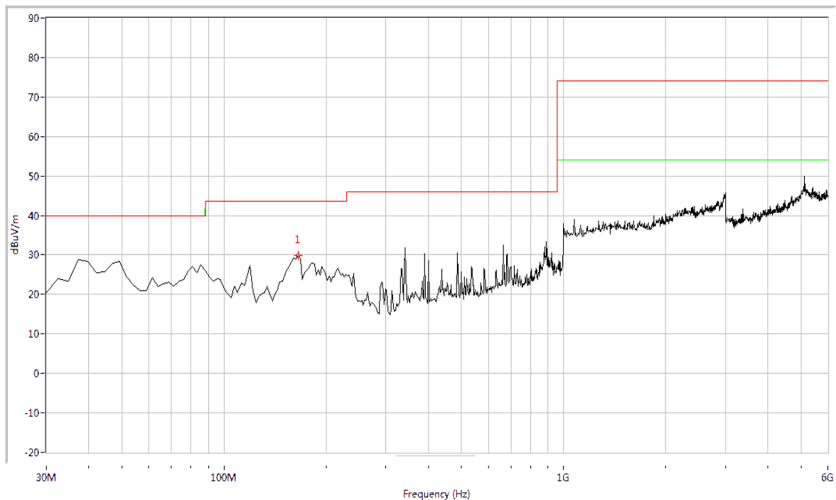
(Plot A: 30MHz – 6GHz, Test Antenna Vertical)
