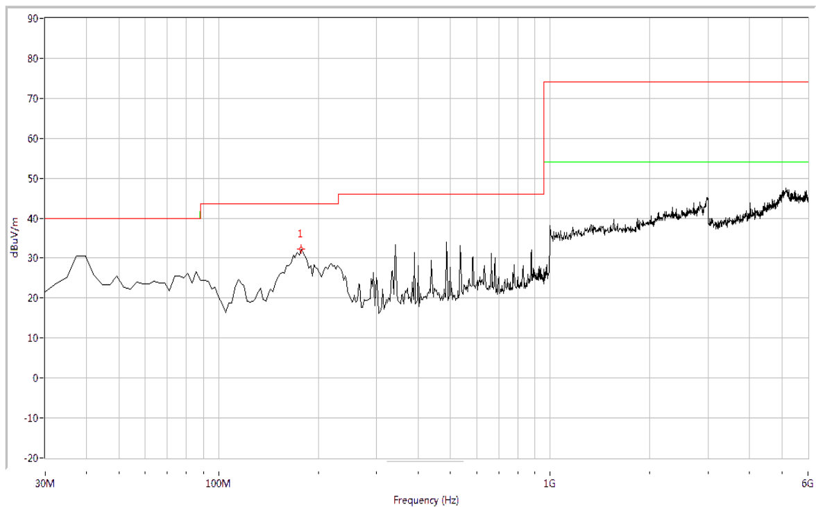
(Plot A: 30MHz – 6GHz, Test Antenna Vertical)
