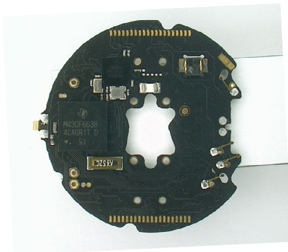
E-module – A-side
