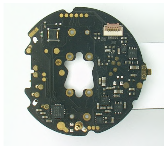
E-module – B-side
