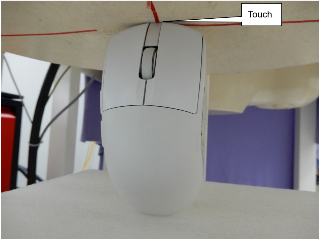
EUT Top
