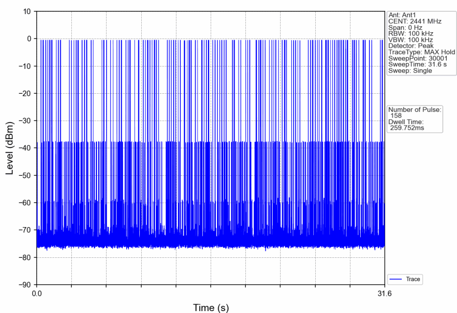
GFSK DH3 HOPP Ant1 NTV
