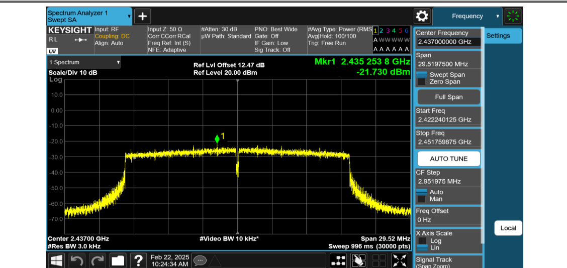
11AX20MIMO-Ant1-2437-PASS
