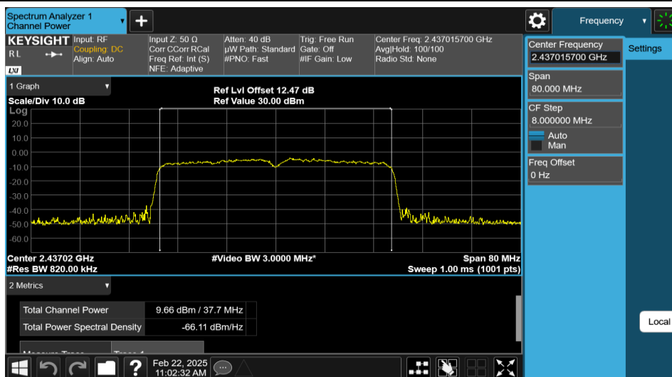
11AX40MIMO-Ant1-2437-PASS
