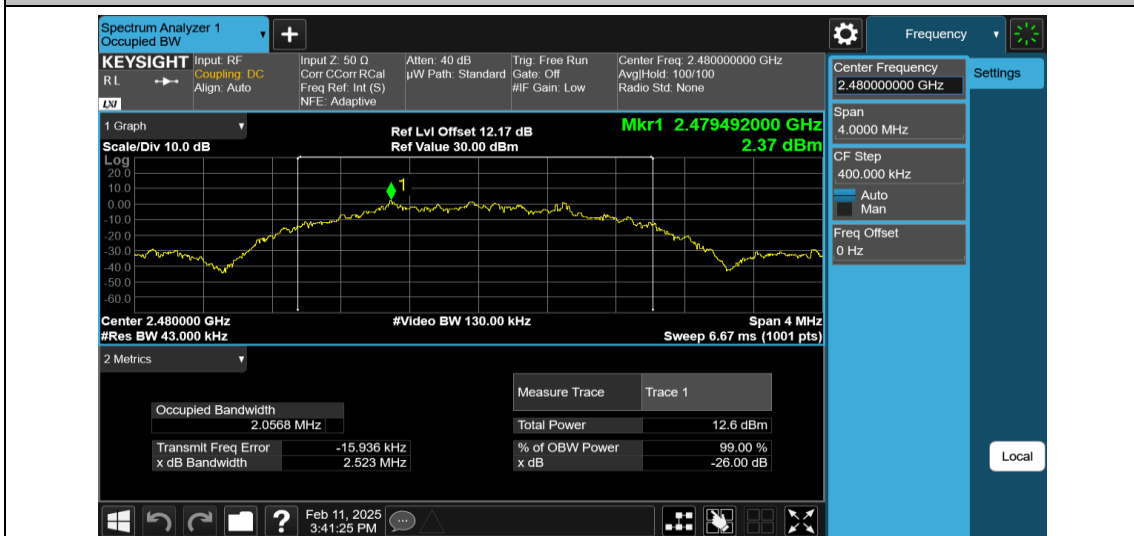
BLE_2M-Ant1-2480
